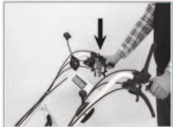
2) Durch Betätigen des rechten oberen Hebels schalten Sie den Fahrtrieb ein.
