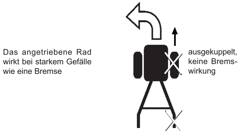
Lenkhilfe rechts bei starkem Gefälle
