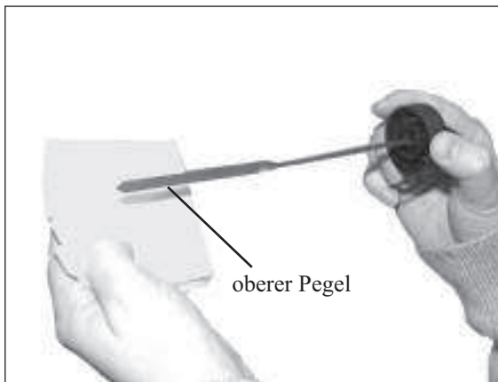
2) Ölmesstab B&S-Motor.
